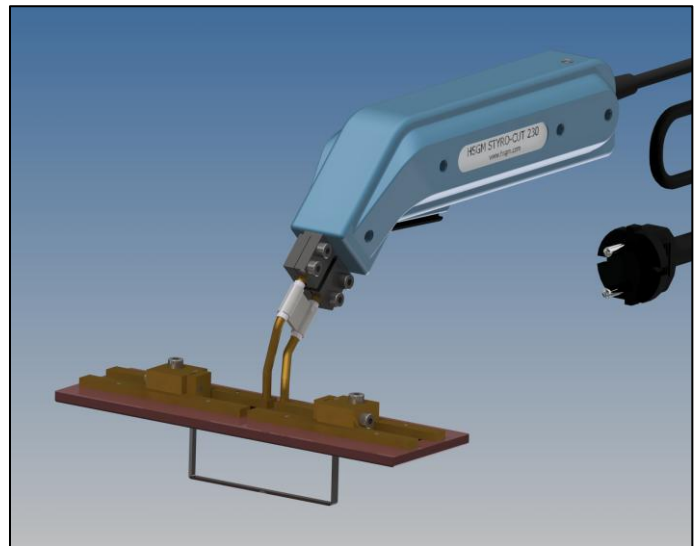
Profilschnittadapter mit HSGM-Styro-Cut-230 (HSGM-Styro-Cut 230 und Schneidband nicht im Lieferumfang enthalten!)
