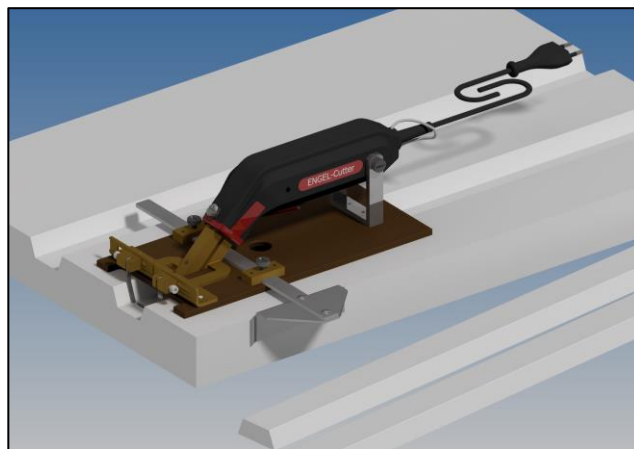
H-A-Adapter mit Engel-Cutter (Engel-Cutter nicht im Lieferumfang enthalten!)
